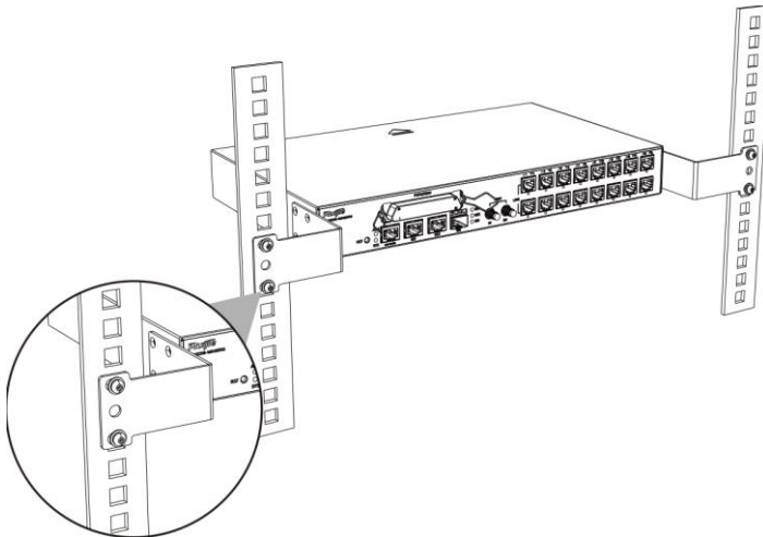
図 3-3 ラックにブラケットを取り付ける
