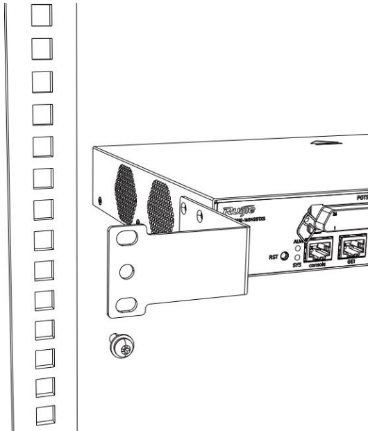
図 3-2 取り付け穴の合わせ方
