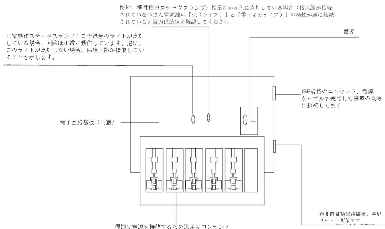
図 C-1 電源避雷器の概要を示す図
